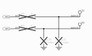
NFC antenna input
